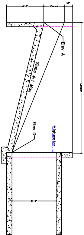
LONGITUDINAL SECTION
